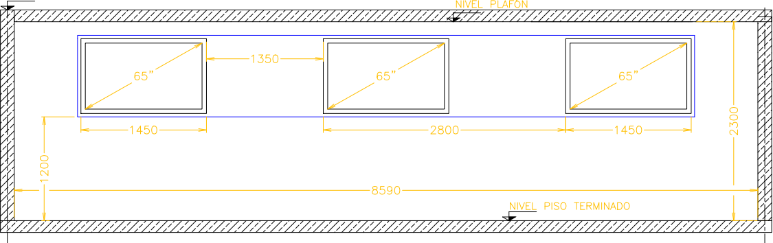
VISTA LATERAL ESCALA 1:60
